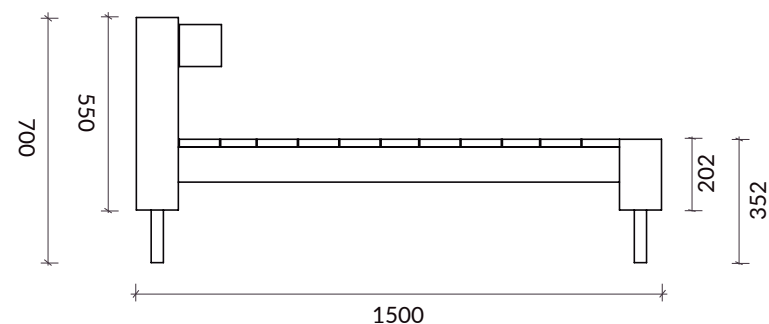
VISTA LATERAL
