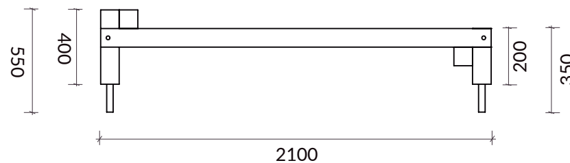
VISTA LATERAL
